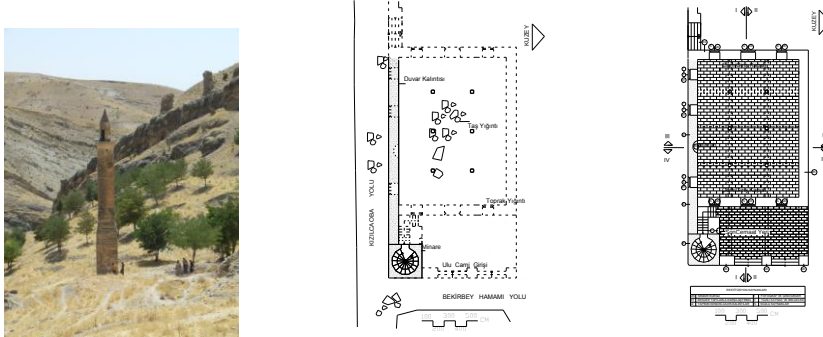
Şekil 1. Ulu Camii Resim ve Planları (Rölöve ve Restitüsyon)
