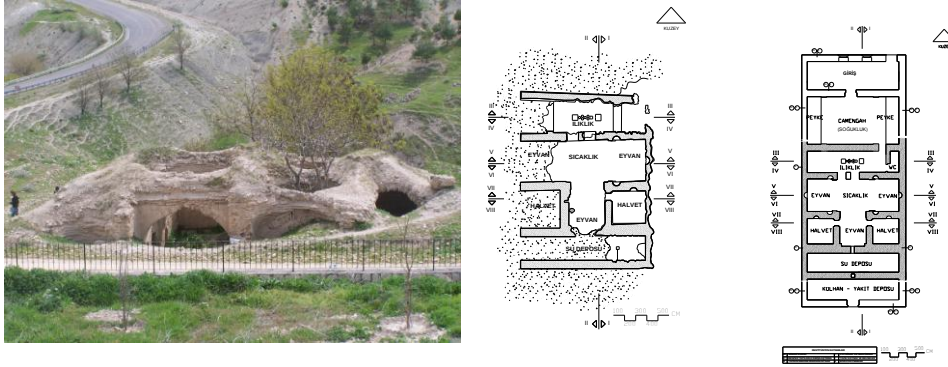
Şekil 5 Meydan Hamamı Resim ve Planları (Rölöve ve Restitüsyon)
